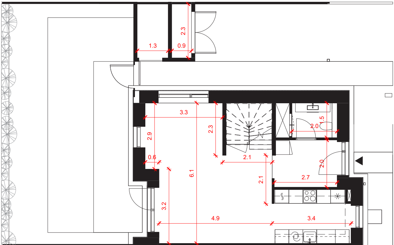
Bolig Nr 13 Stueplan BØGEN 5
