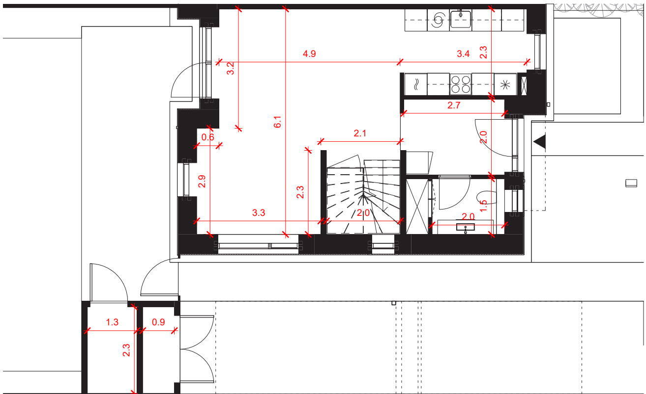
Bolig Nr 22 Stueplan FYRREN 5
