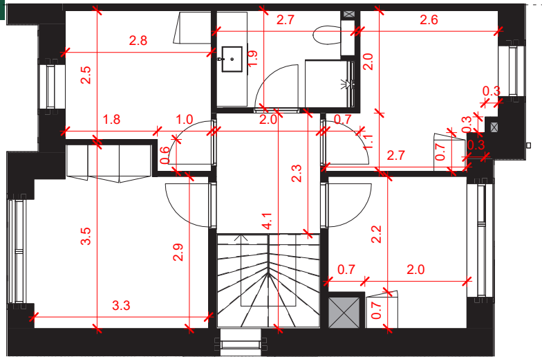
Bolig Nr 22 1.sal
