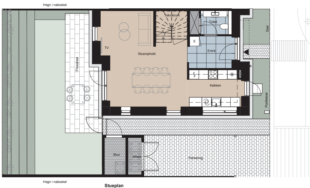
Stueplan
