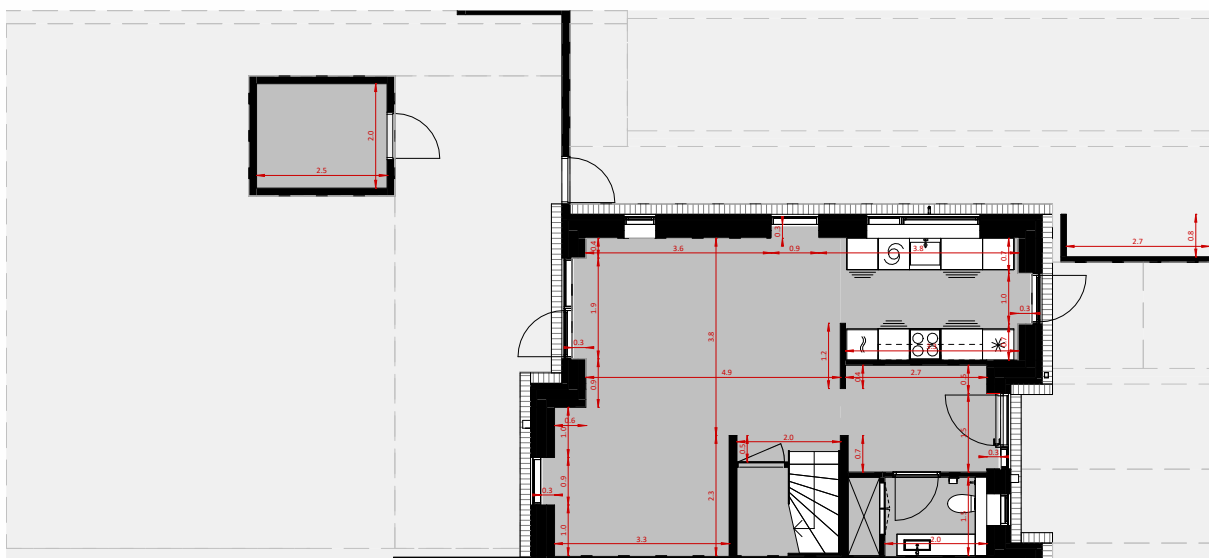
Stueplan
